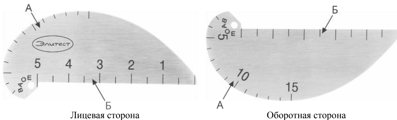
Рисунок 1 – Общий вид универсального шаблона сварщика УШС-1 ЭЛИТЕСТ А, Б – измерительные шкалы
