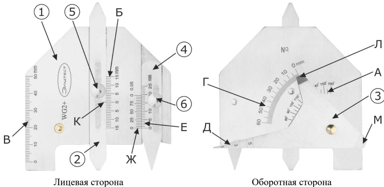
Рисунок 1 – Общий вид измерительного шаблона сварщика WG2+ ЭЛИТЕСТ 1 – основание; 2, 3, 4 – измерительные движки; 5, 6 – стопорные устройства движков (2) и (4) соответственно; А, Б, В, Г, Д, Е – измерительные шкалы; Ж – нониус шкалы (Е); К, Л, М – контрольные риски-индексы шкал (Б), (Г) и (А) соответственно
