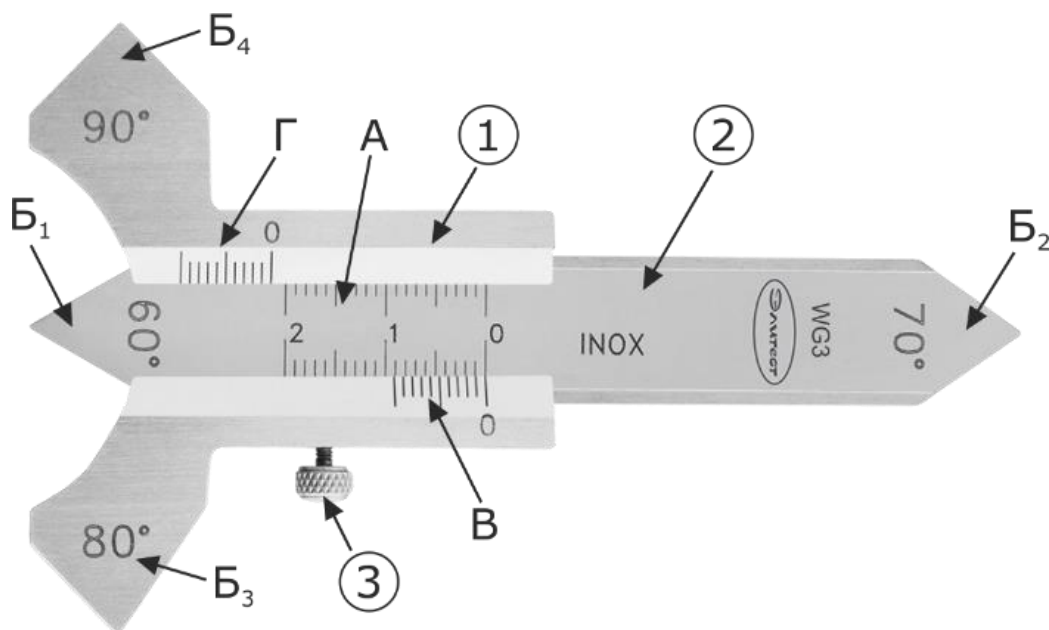
Рисунок 1 – Общий вид измерительного шаблона сварщика WG3 нониусный ЭЛИТЕСТ
