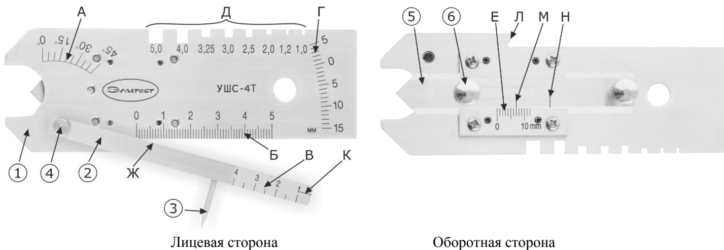
Рисунок 1 – Общий вид универсального шаблона сварщика УШС-4Т ЭЛИТЕСТ
